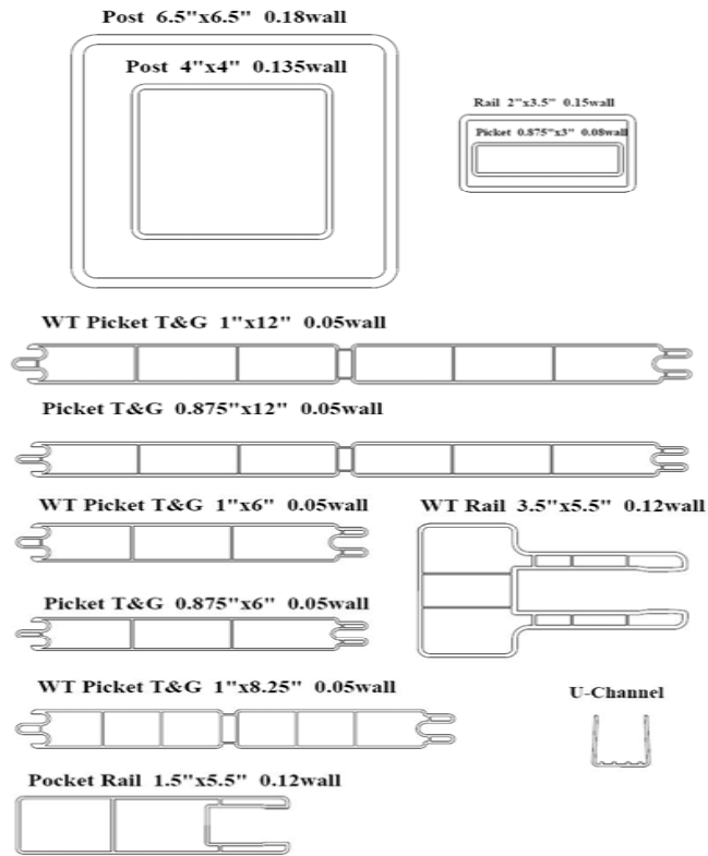
WindTamer Profiles
